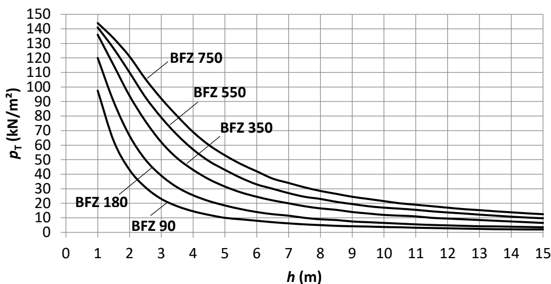
Bild C.1: Bodenspannungen p_T infolge von Flugzeugverkehrslasten
